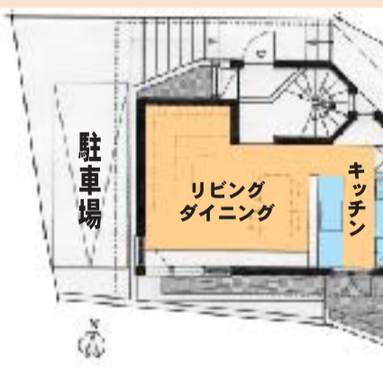
1階平面図
